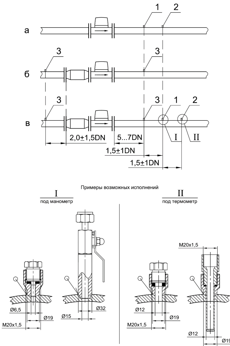
Рисунок Г.5 – «Врезка» штуцеров в ЭТ при монтаже ПП ИРВИС-Ультра-Пп
