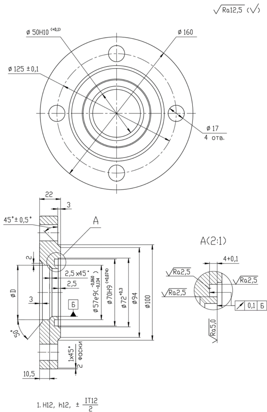
Рисунок Г.6 – Конструкция, габаритные и присоединительные размеры ответного фланца ИРВИС-Ультра-Пп-16-DN50
