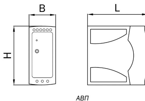
Рисунок Б.2 - Габаритные и присоединительные размеры БИП ИРВИС-Ультра-Пп-16
